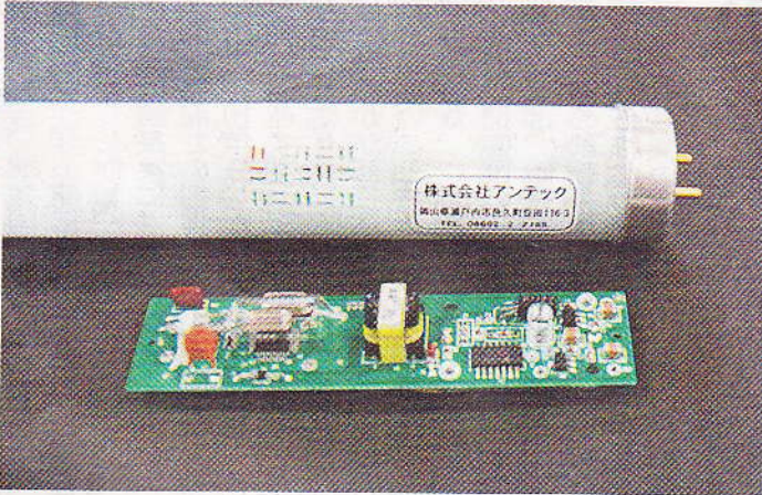
アンテックが開発した火災センサー内蔵型の LED蛍光灯。手前がセンサー付きの基板
